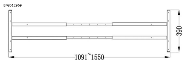
Konsolit ja pitkittäistuet pöytäkanen alla
